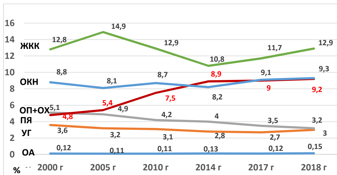
Рис. 1. Динамика послеоперационной летальности при острых заболеваниях органов брюшной полости в России (2000 – 2018 гг.).
