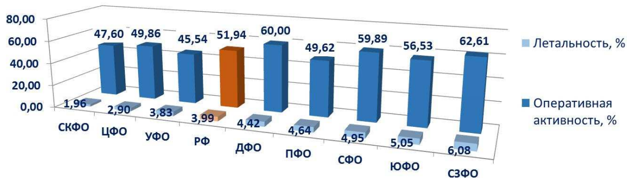
Рис. 3. Соотношение оперативной активности и госпитальной летальности при острой спаечной кишечной непроходимости.
