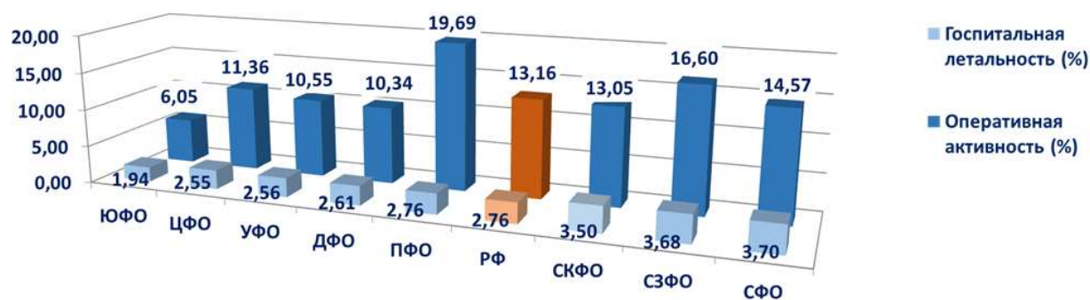
Рис. 6. Соотношение госпитальной летальности и оперативной активности при остром панкреатите ( r=0,63 ; p=0,004 ).
