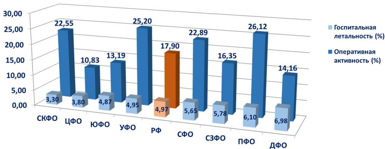
Рис. 4. Соотношение госпитальной летальности и оперативной активности при гастродуоденальных язвенных кровотечениях ( r=0,54 ; p=0,02 ).
