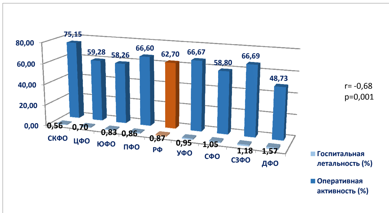
Рис. 5. Соотношение госпитальной летальности и оперативной активности при остром холецистите.
